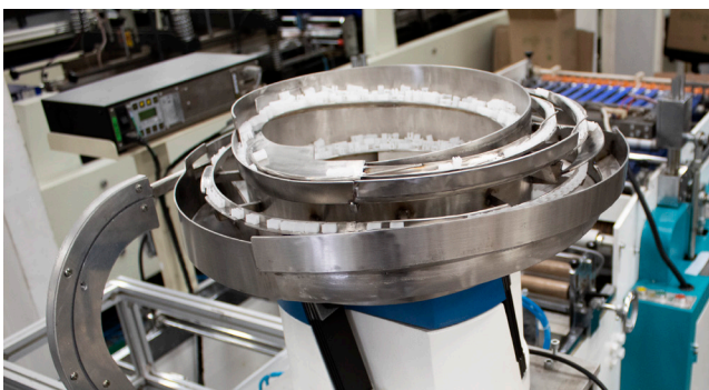
● Aplicador de Slider
